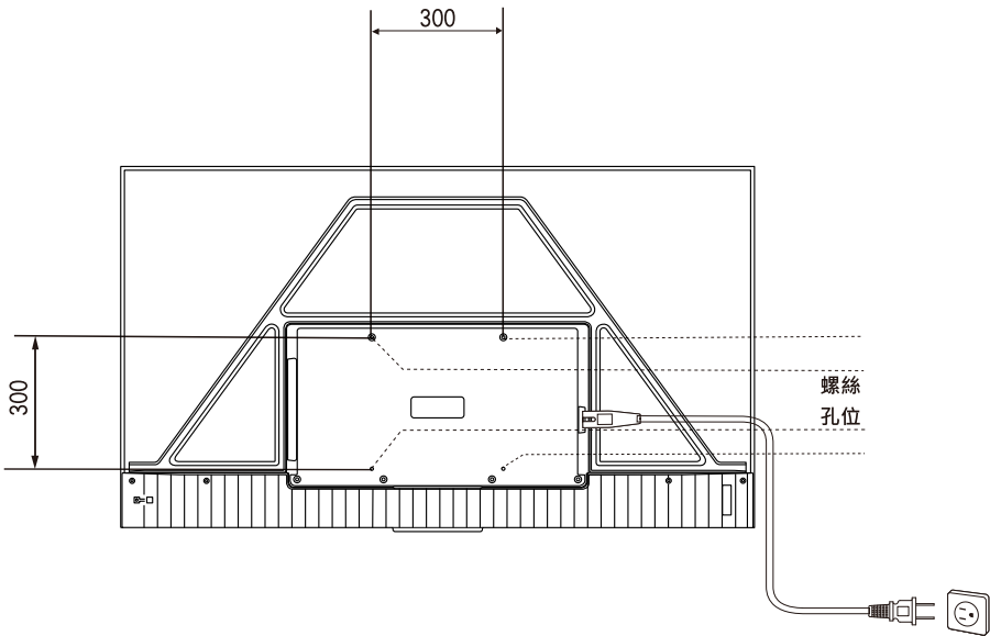
壁掛架示意圖（50/55/65吋）
