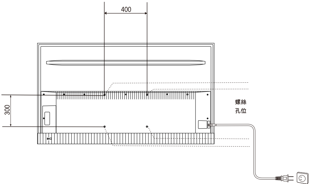
壁掛架示意圖（75吋）
