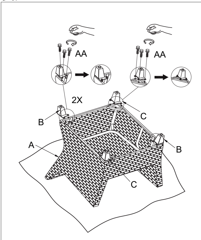
步驟 #4
