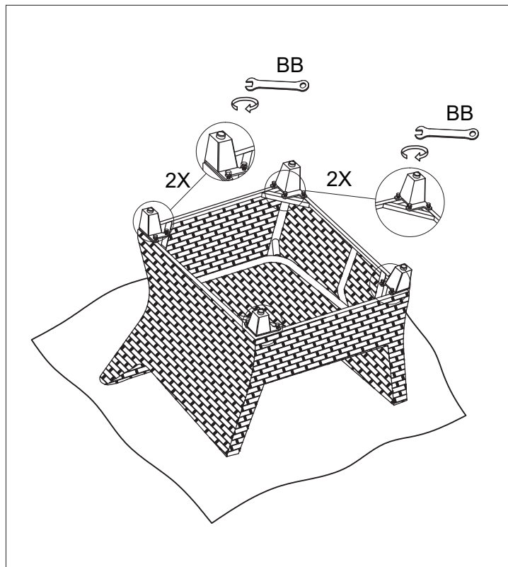
步驟 #5
